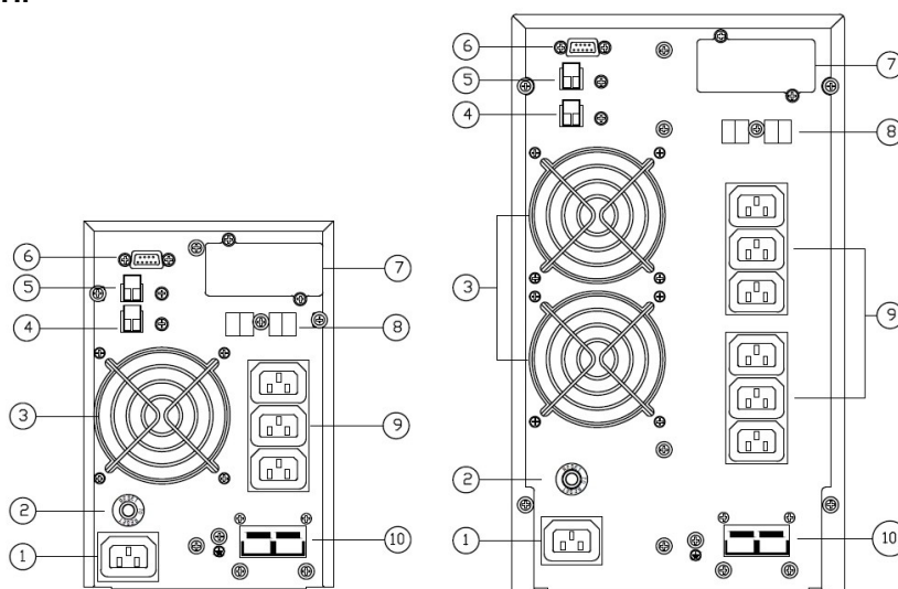
ИБП 1 кВА
