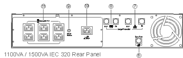
Задняя панель моделей 1100 и 1500
