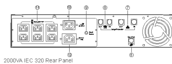
Задняя панель модели 2000
