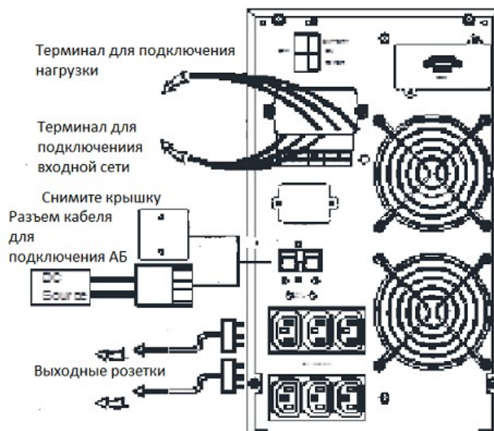
Рис. 3-3 Схема подключения ИБП 1102-1103 (L)
