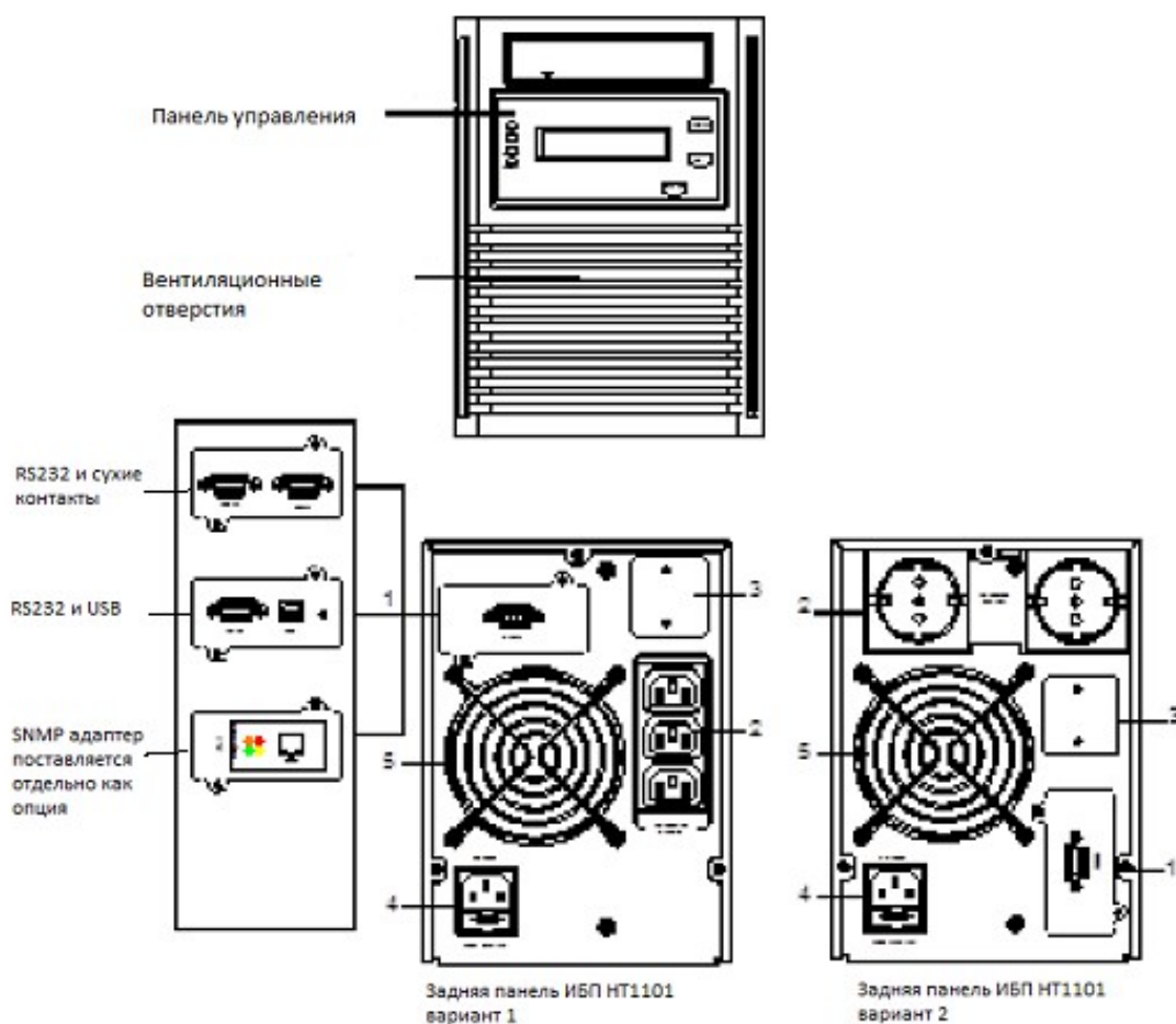
Рис. 2-2 Возможные конфигурации задней панели ИБП HT1101
