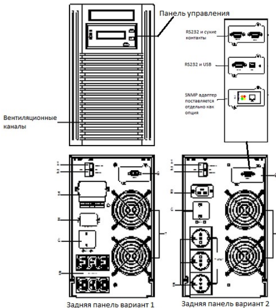
Рис 2-3 HT1102&HT1103 Передняя панель и два варианта задней панели.
