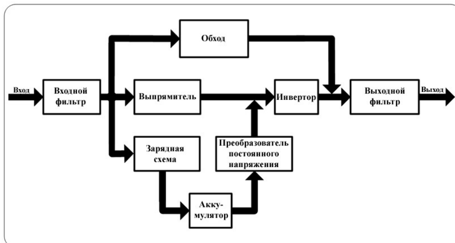
Рис. 2-4 Схема работы ИБП серии HT11
