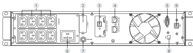
Вид сзади: ИБП ИМПУЛЬС ФРИСТАЙЛ 1000 ВА, 1500 ВА и 2000 ВА
